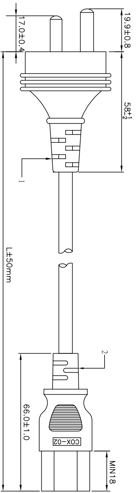
CONNECTOR:COX-02
